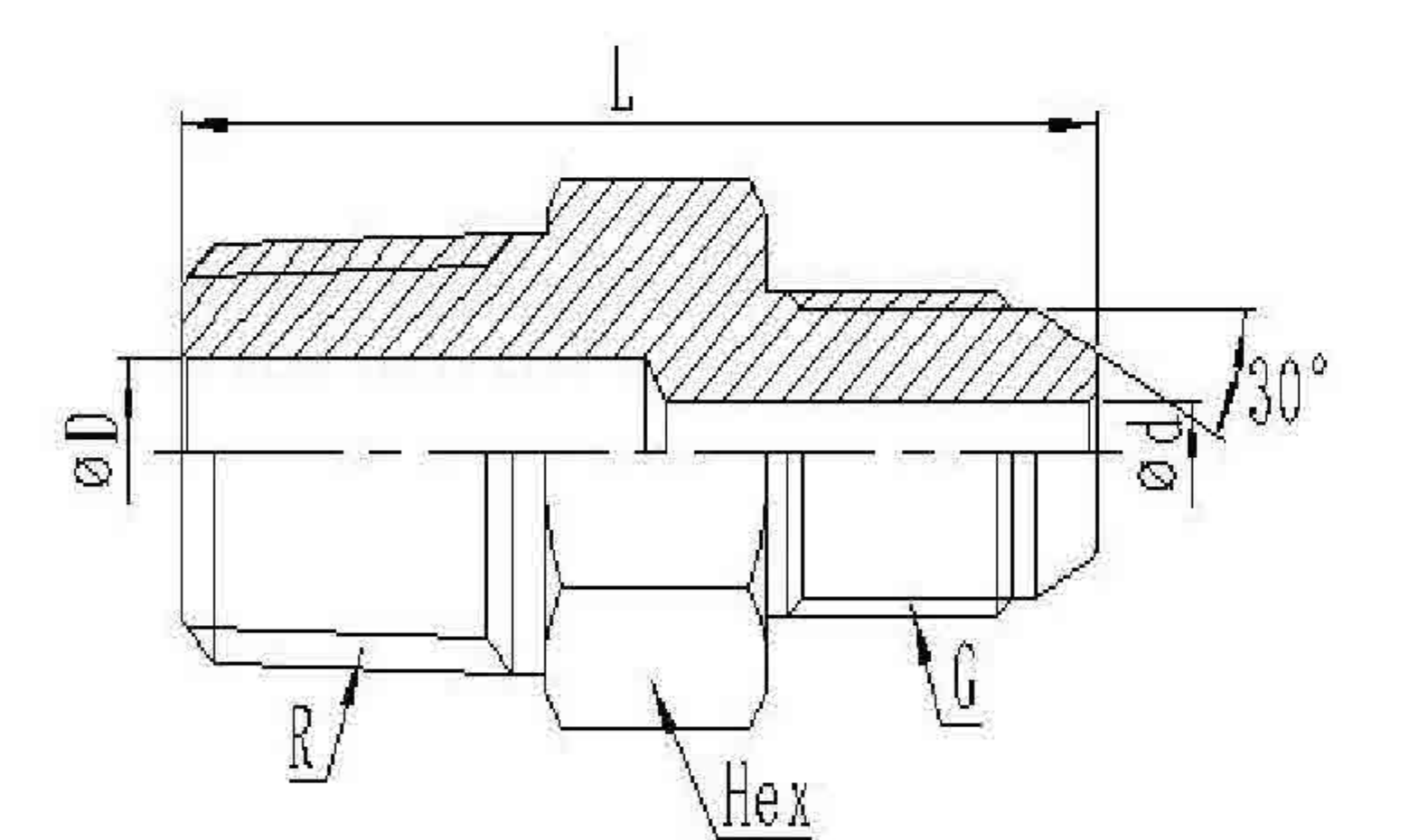
1013R
