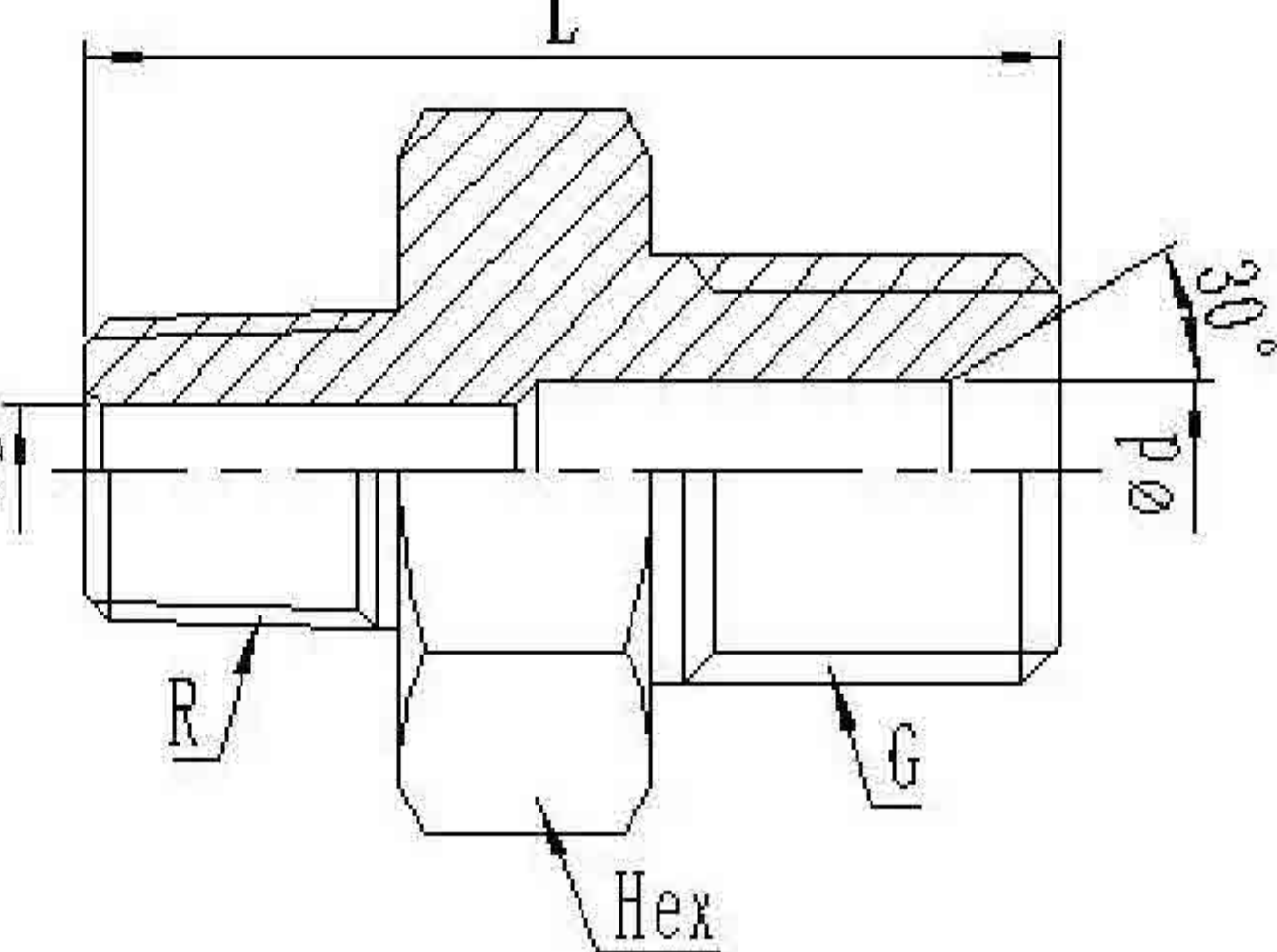
1009R
