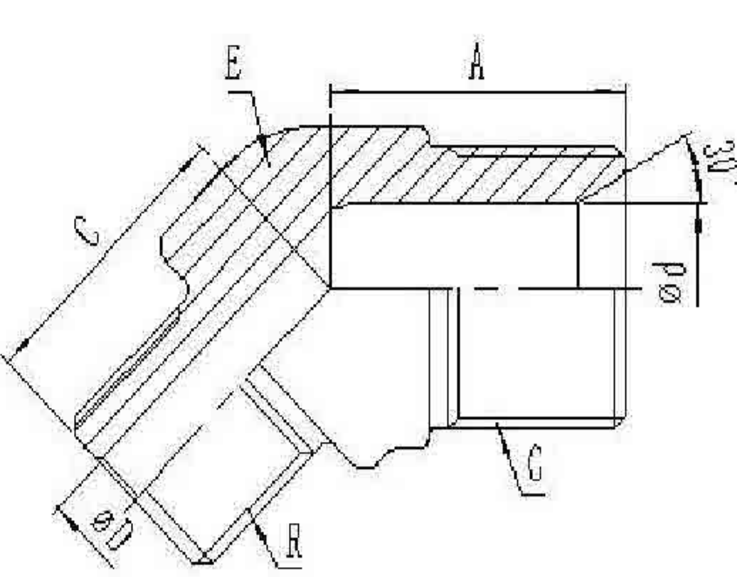
1036S
