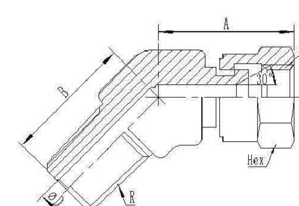
1036S
