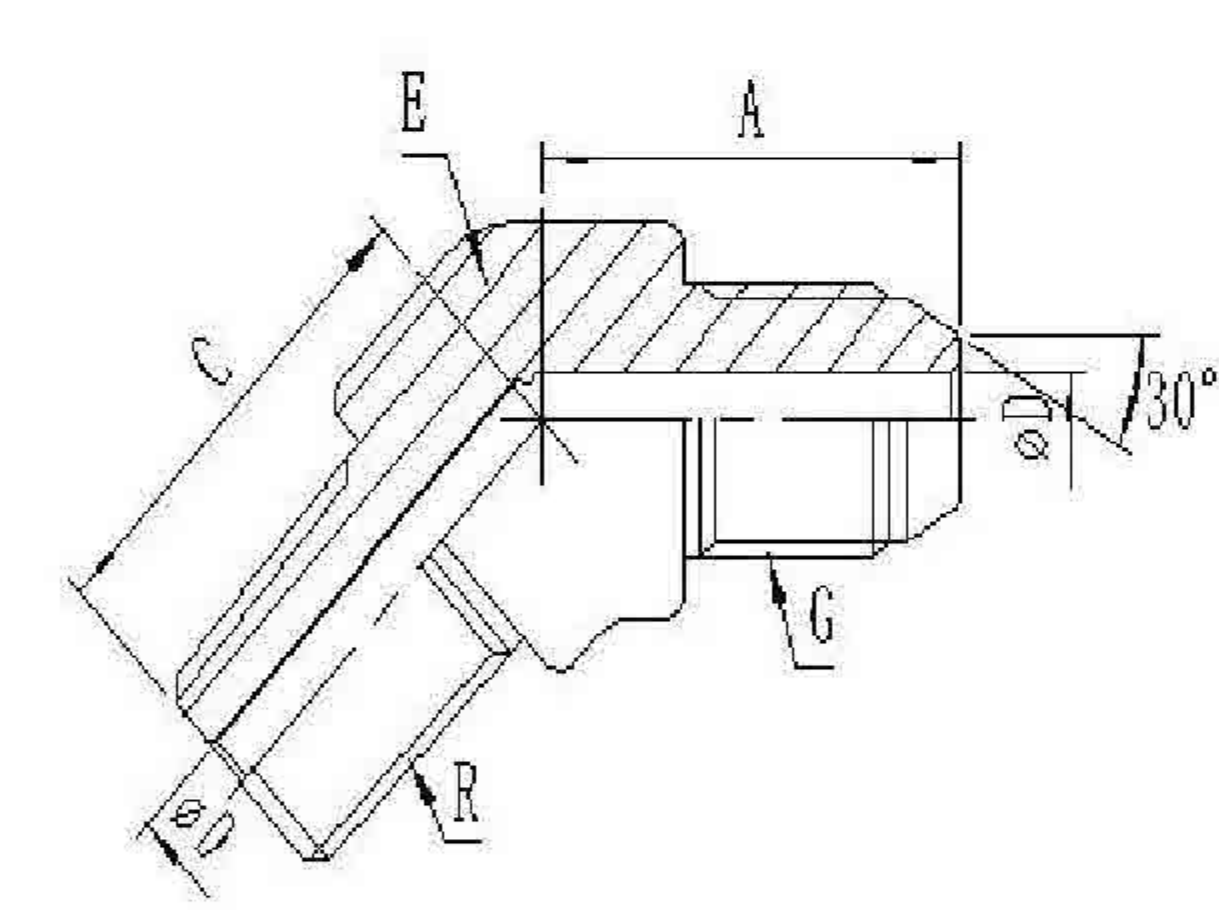
45° ELBOW 1035
