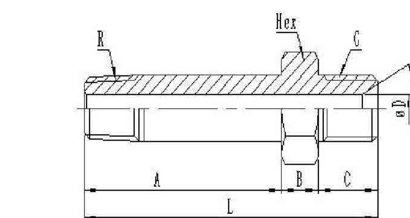
1009L
