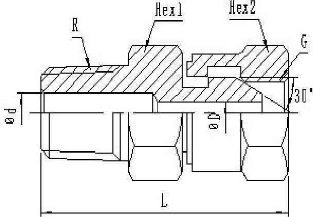
1006R
